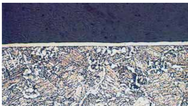
Nitrocarburierter C15, VS = 15.1-15.4 my, Oberflächenhärte als Mittelwert = 492 HV 0.3
