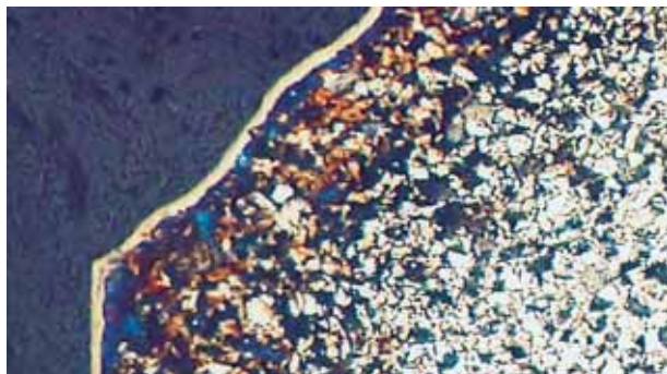
Rheinnitrierter 16 MnCr 5, VS = 12-15 my, NHT = 0.544 mm, Oberflächenhärte als Mittelwert = 632 HV 0.5
